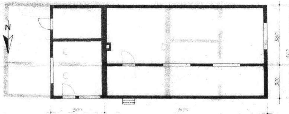
Grundriß
